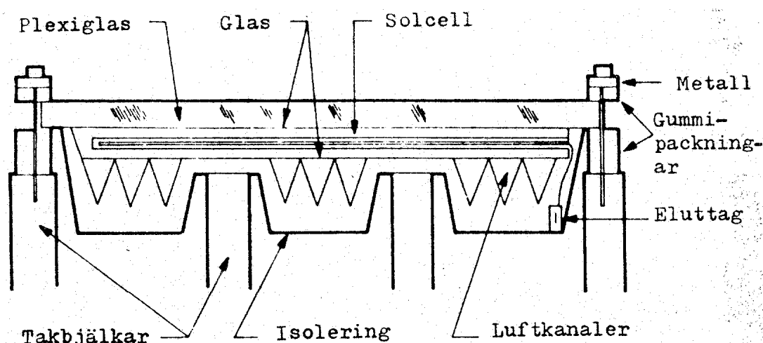
Fig. 3.4.3.5 Tak- eller vägghängd panel med solceller inbyggda i en solfångare
