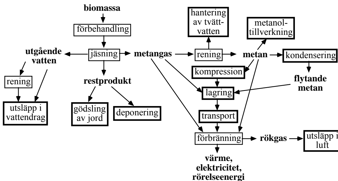
Fig. 4.14.3 "Riskschema" över metanjäsnings. Varje steg som kan innebära en möjlig risk betecknas med en "fet" låda.
