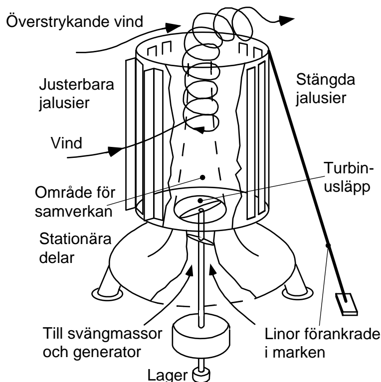
Fig. 5.4.3 Tomadokraftverk
