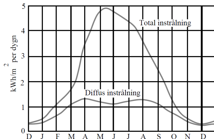
Fig. 3.1.c Genomsnittlig instrålning mot en horisontell yta. Totalvärde och andel diffust ljus
