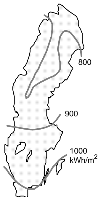
Fig. 3.2 Totalt infallande solenergi per år i Sverige
