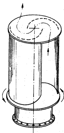
Fig. 5.4.2 a Savonius-turbin
